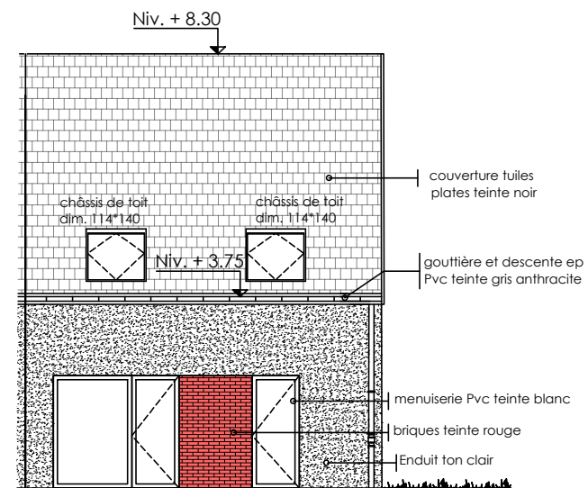
Façade Arrière
